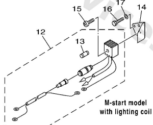
RECTIFIER KIT
