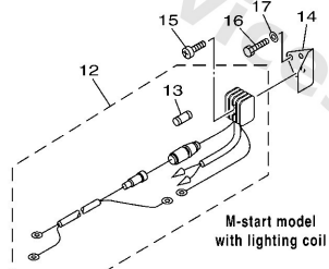
RECTIFIER KIT
